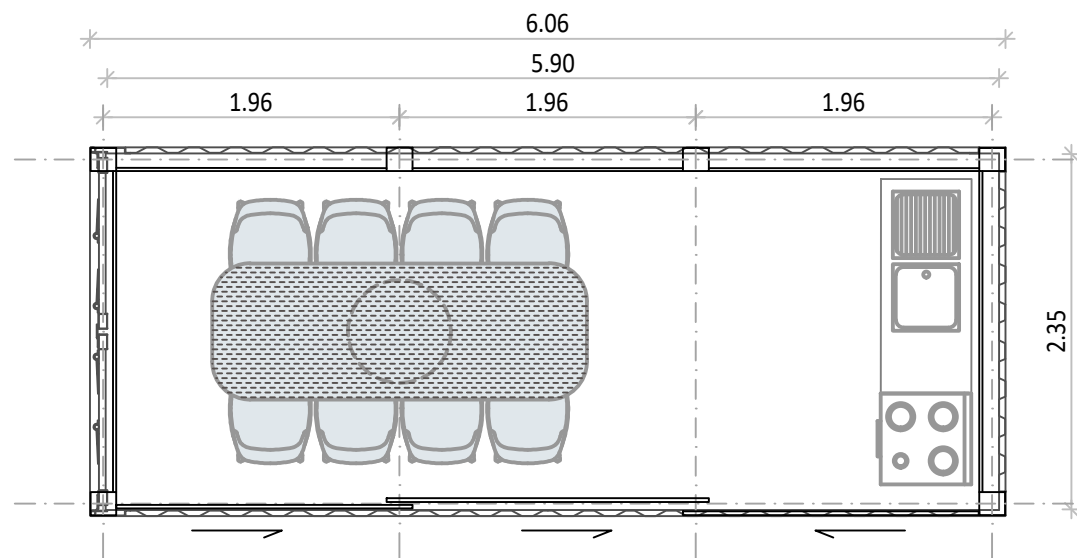
PERGOLA + LETNA KUHINJA
