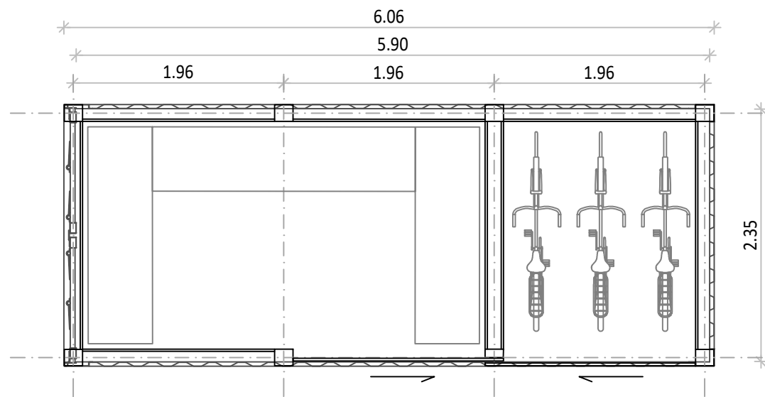
VRTNA LOPA + KOLESARNICA
